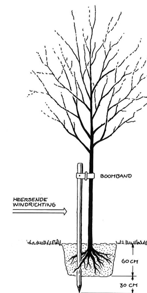
Plaatsing boompaal ten opzichte van overheersende windrichting.
