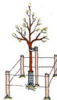
Voorbeeld van aanbrengen afrastering op afstand om vraat door vee onmogelijk te maken.
