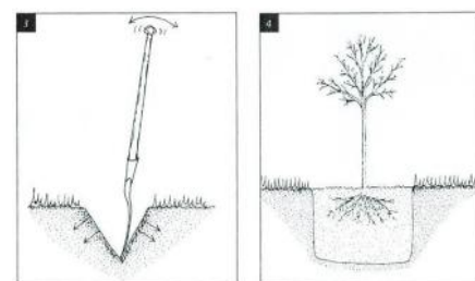
Voorbeeld maken van plantgat. Links is fout, rechts is goed.
